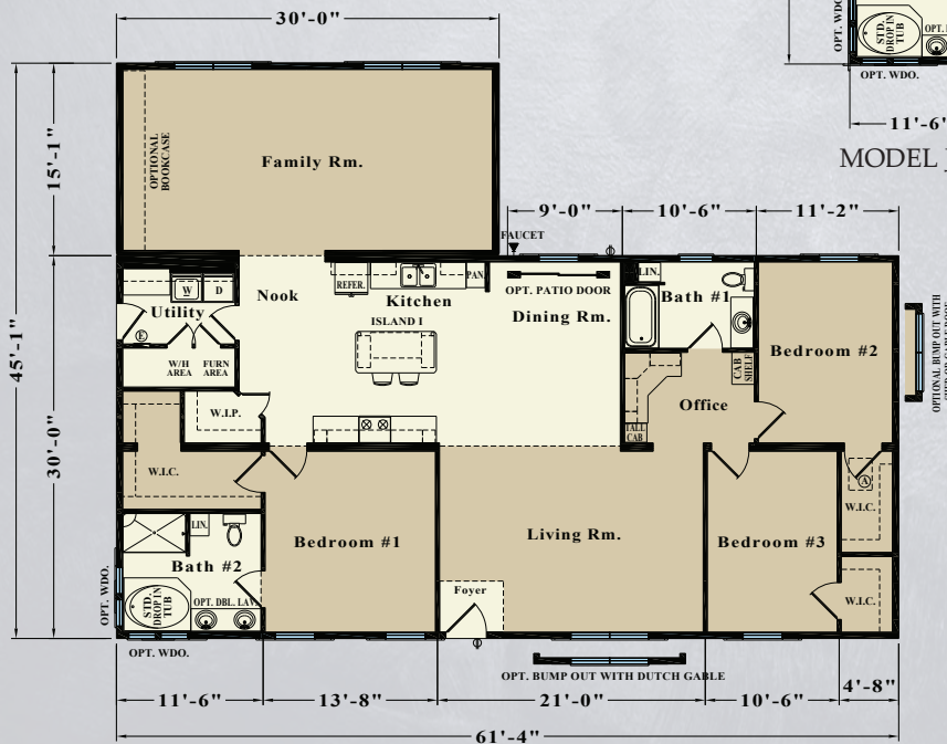
MODEL EJ31A - 2,290 S.F.
